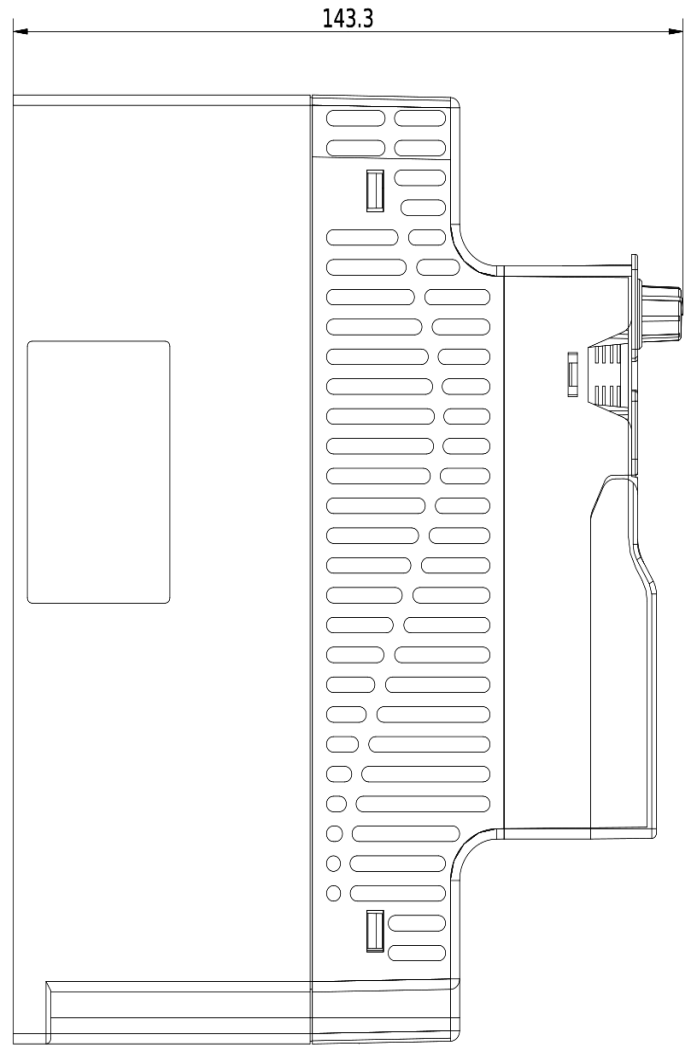
Rozmerový výkres V800 - 4kW 4T0040
