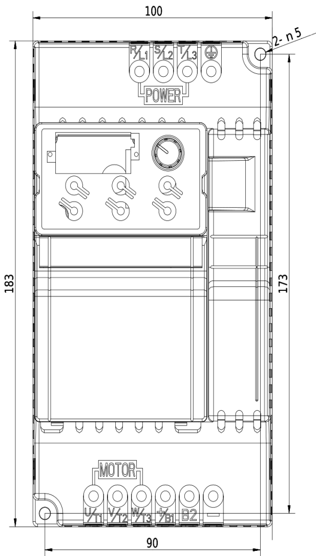
Rozmerový výkres V800 - 4kW 4T0040
