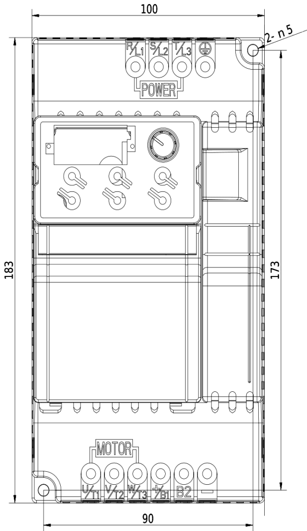
Rozmerový výkres V800 - 5,5kW 4T0055
