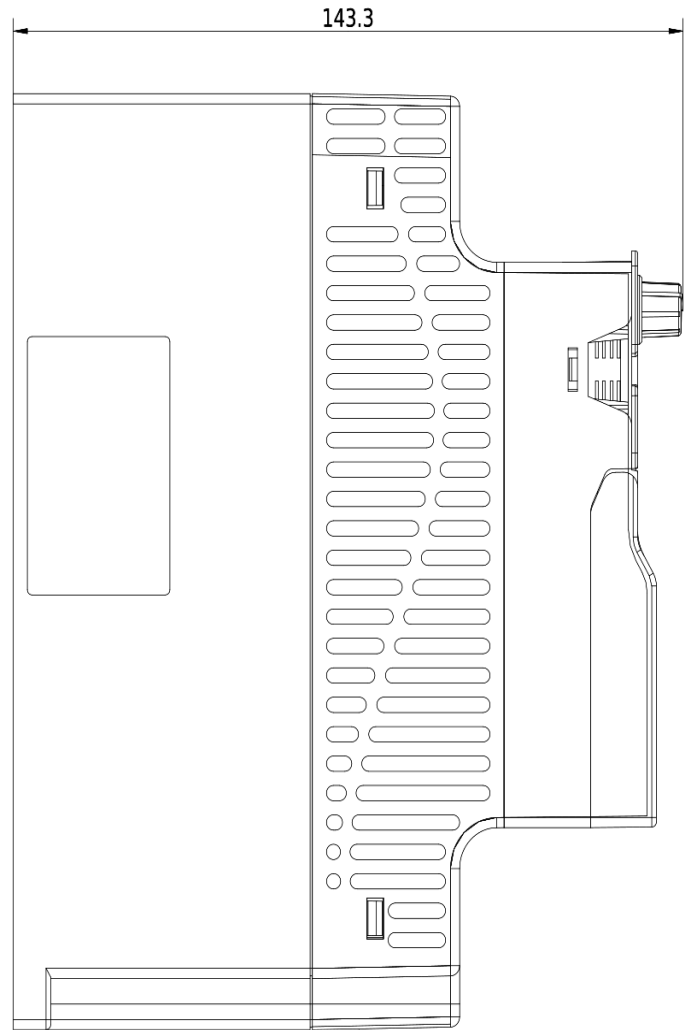
Rozmerový výkres V800 - 5,5kW 4T0055
