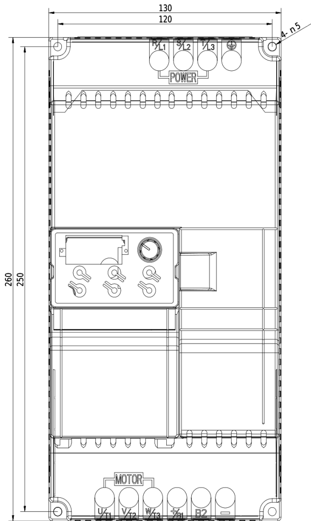
Rozmerový výkres V800 - 7,5kW 4T0075
