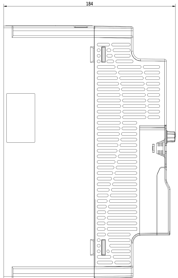
Rozmerový výkres V800 - 7,5kW 4T0075
