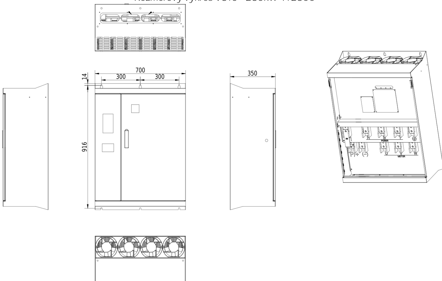
Rozmerový výkres V810 - 280kW 4T2800
