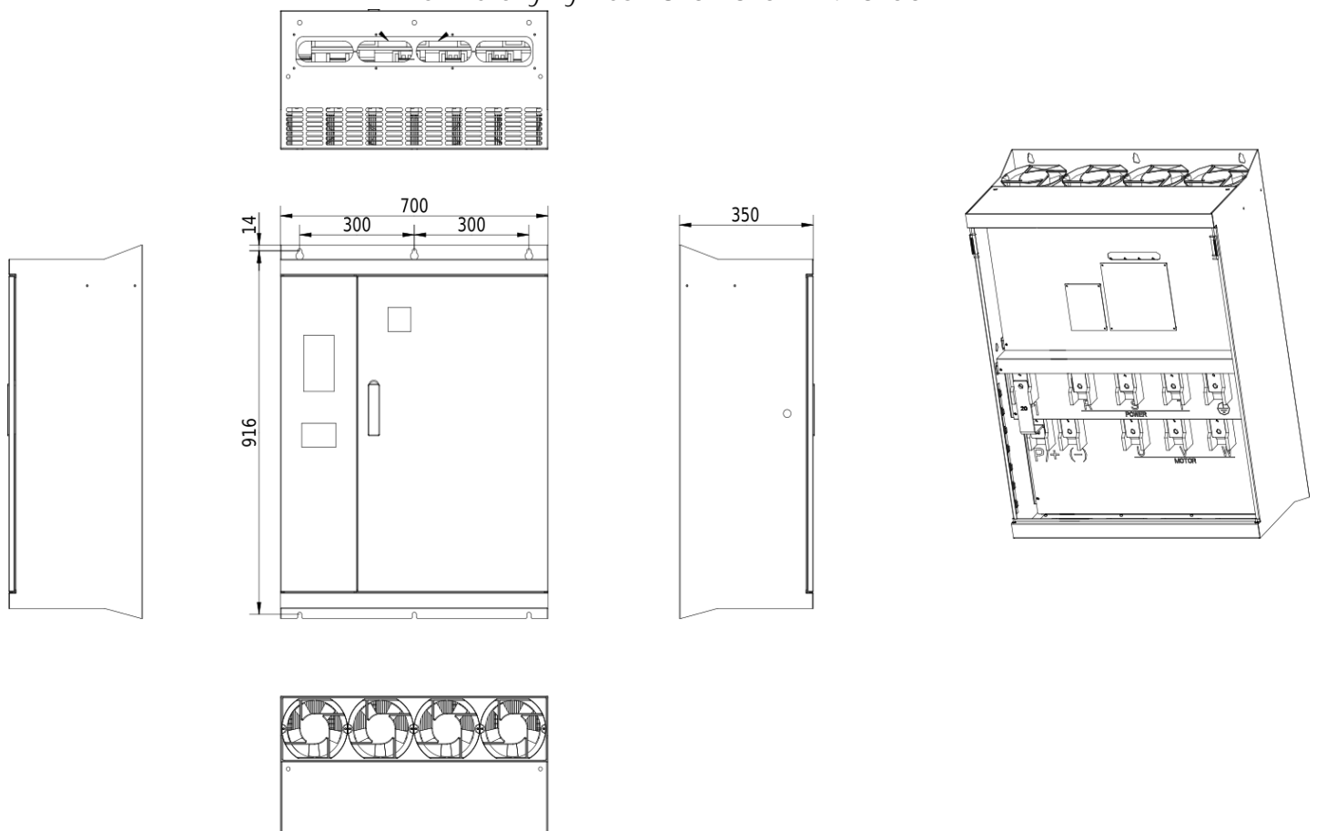
Rozmerový výkres V810 - 315kW 4T3150
