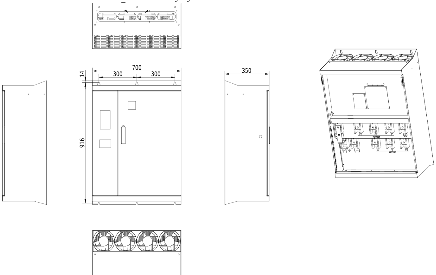
Rozmerový výkres V810 - 355kW 4T3550
