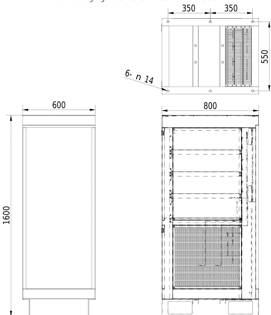
Rozmerový výkres V810 - 400kW 4T4000
