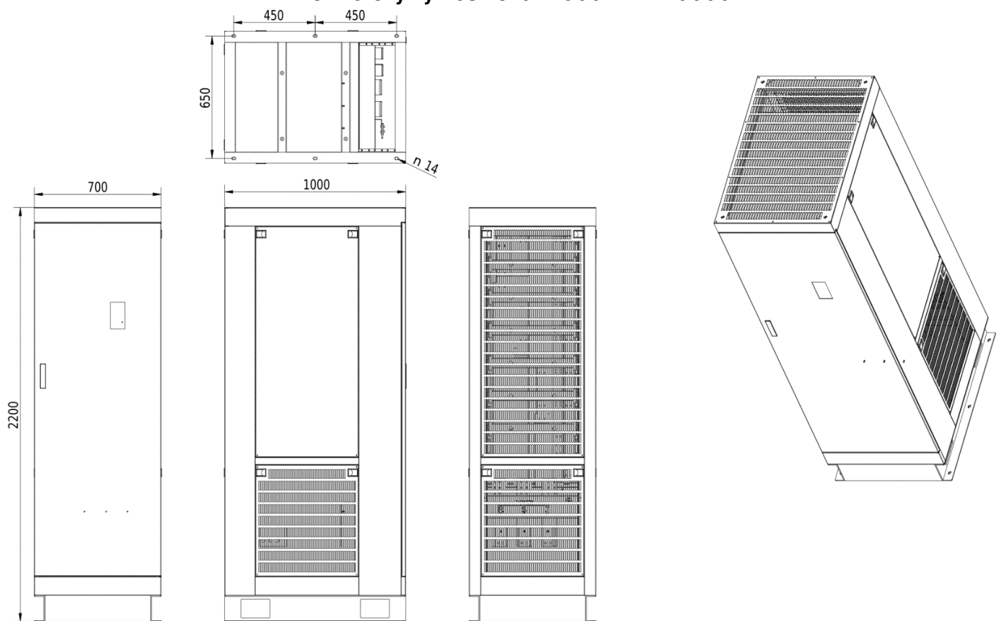
Rozmerový výkres V810 - 1000kW 4T10000
