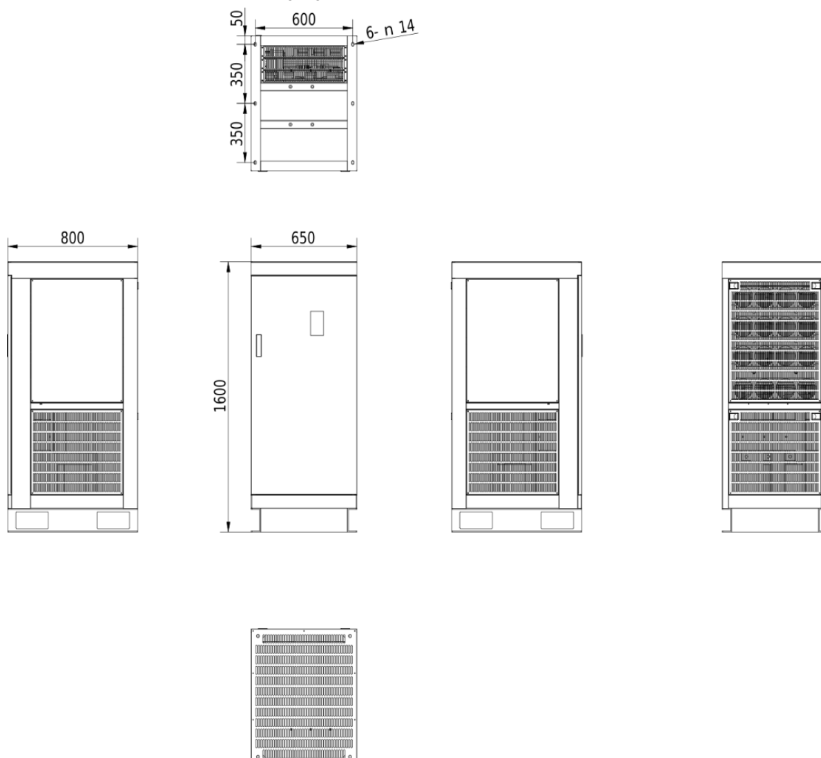
Rozmerový výkres V810 - 710kW 4T7100
