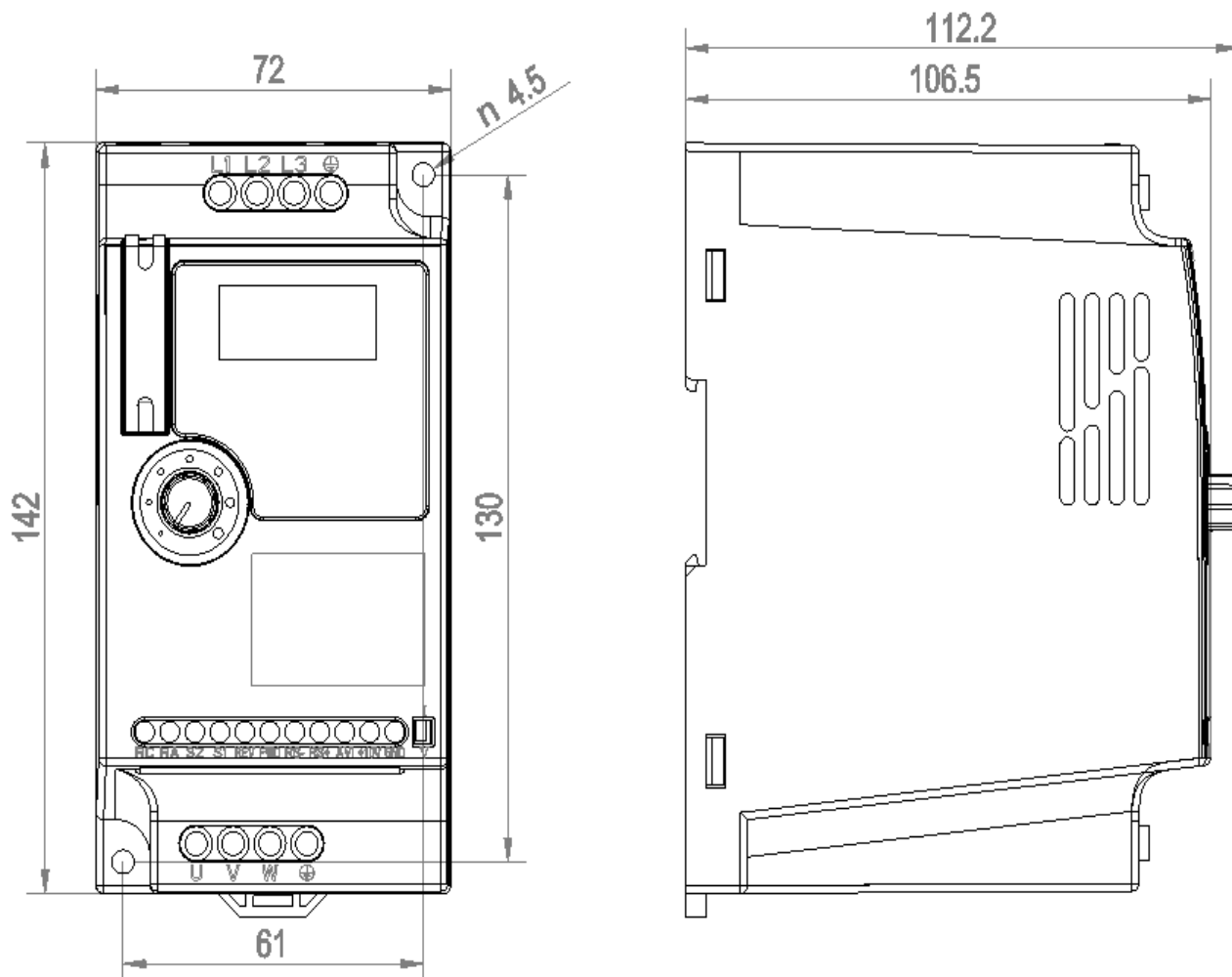
Rozmerový výkres A550 PLUS - 1,5kW 4T0015
