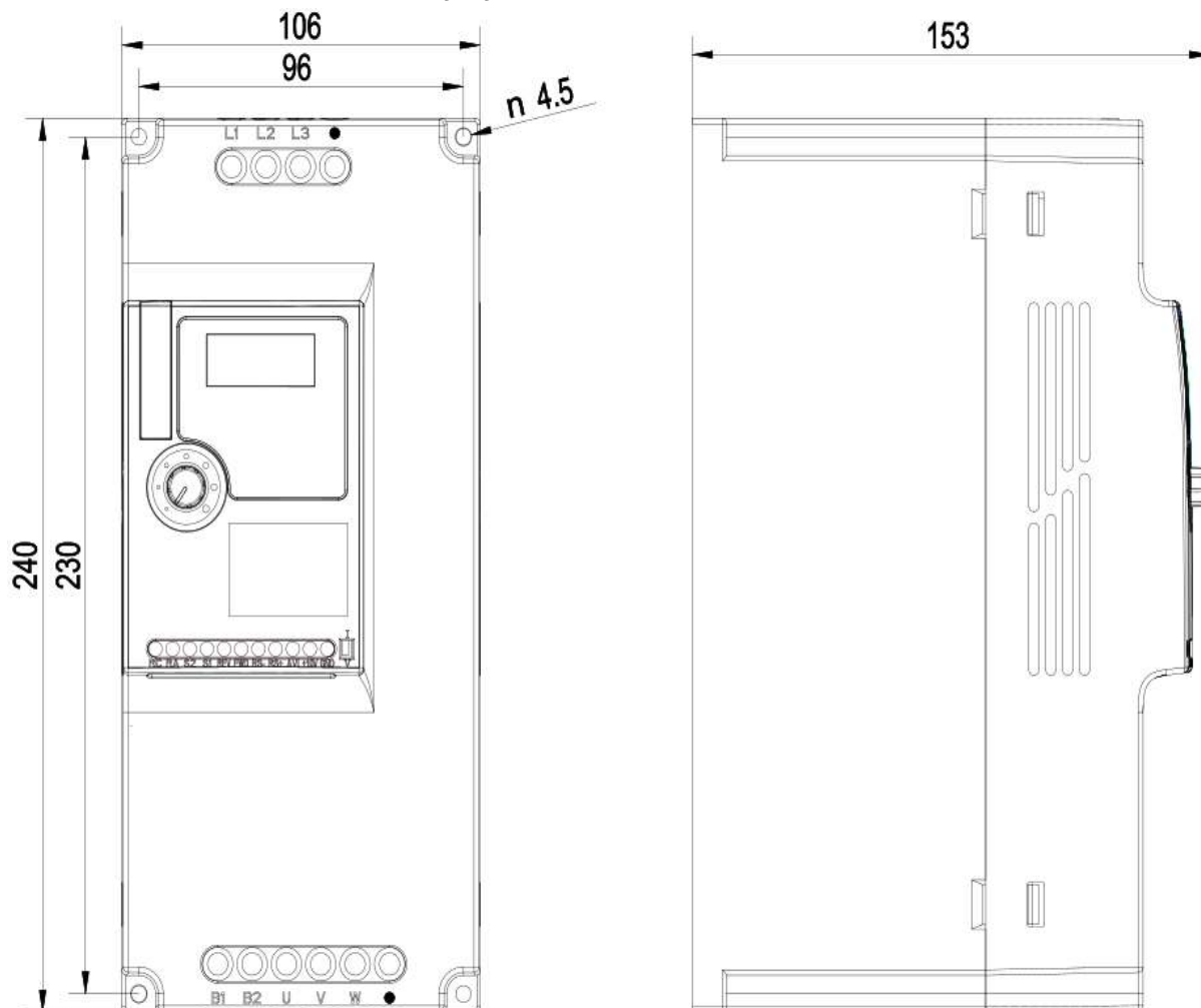
Rozmerový výkres A550 PLUS - 7,5kW 4T0075
