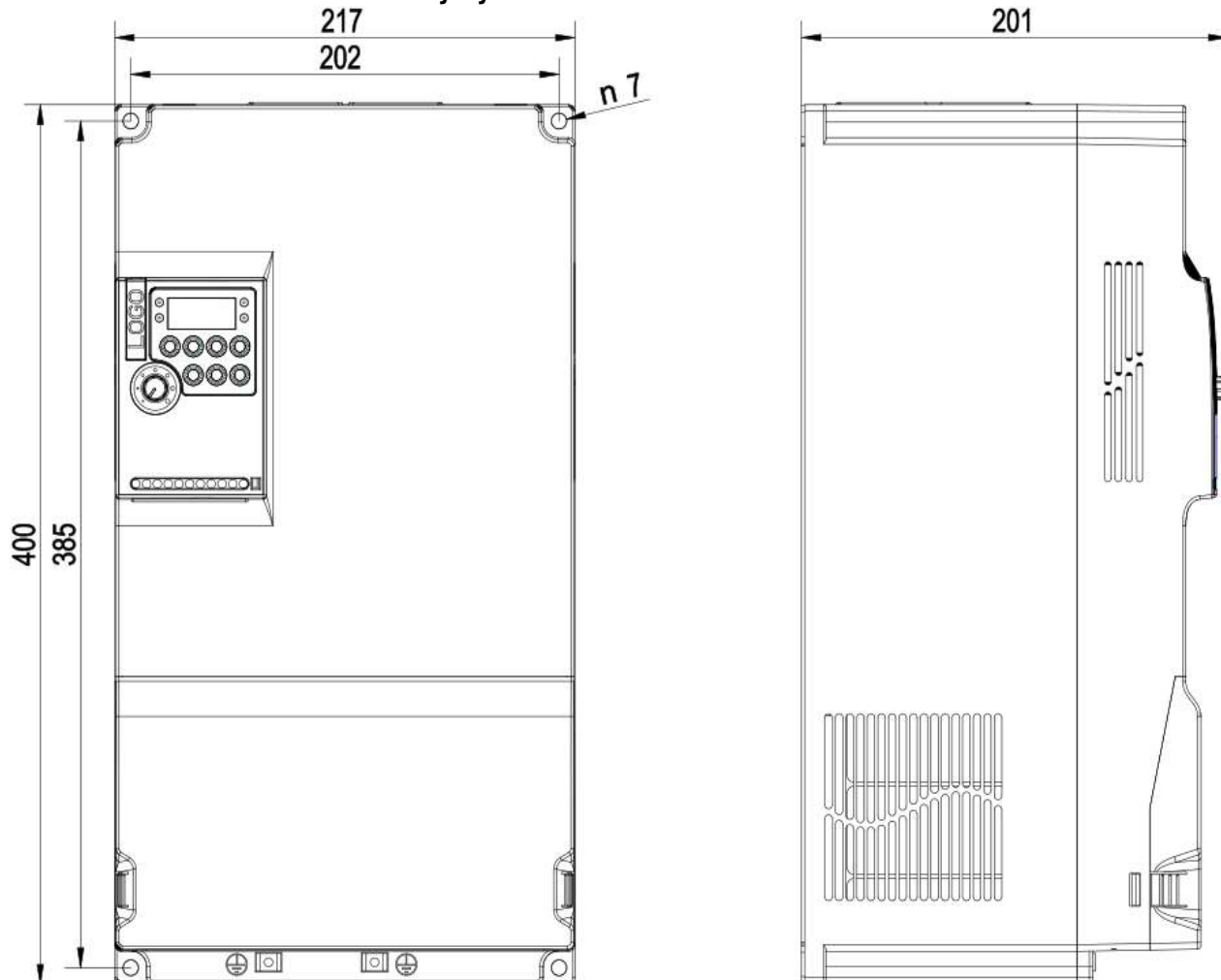
Rozmerový výkres A550 PLUS - 30kW 4T0300
