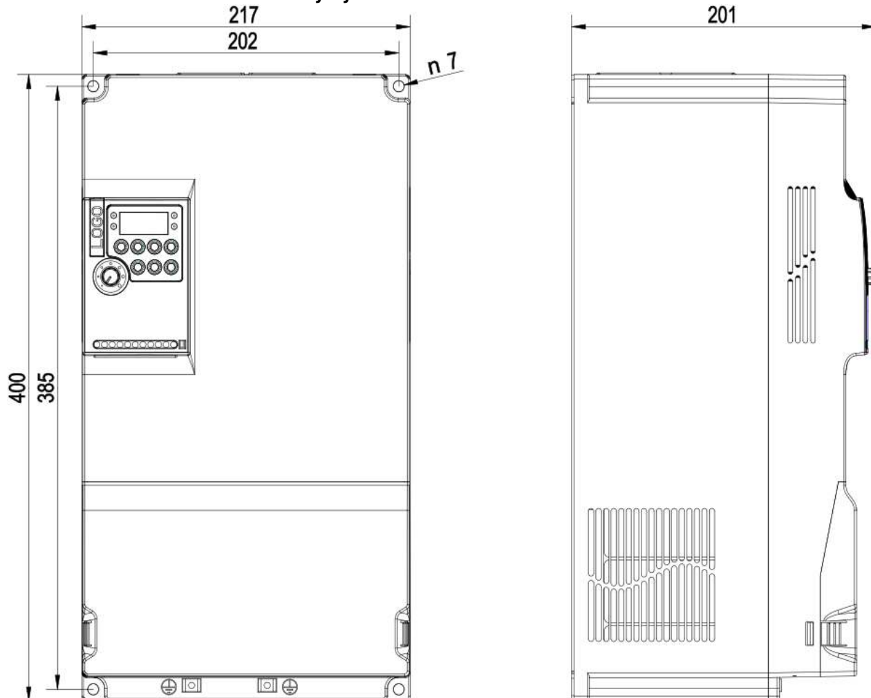
Rozmerový výkres A550 PLUS - 37kW 4T0370
