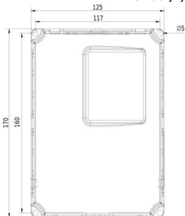
Rozmerový výkres V810 - 0,4kW 2S0004
