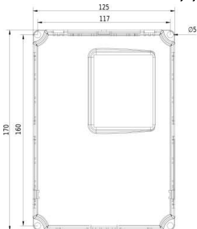
Rozmerový výkres V810 - 0,4kW 4T0004
