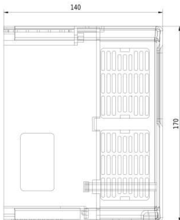
Rozmerový výkres V810 - 0,75kW 4T0007
