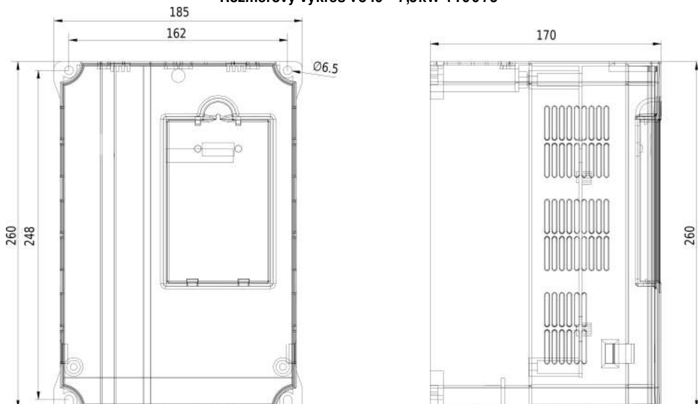
Rozmerový výkres V8 10 - 7,5kW 4T0075
