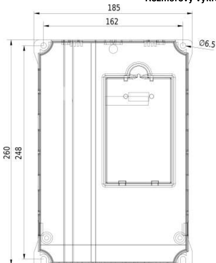
Rozmerový výkres V810 - 11kW 4T0110
