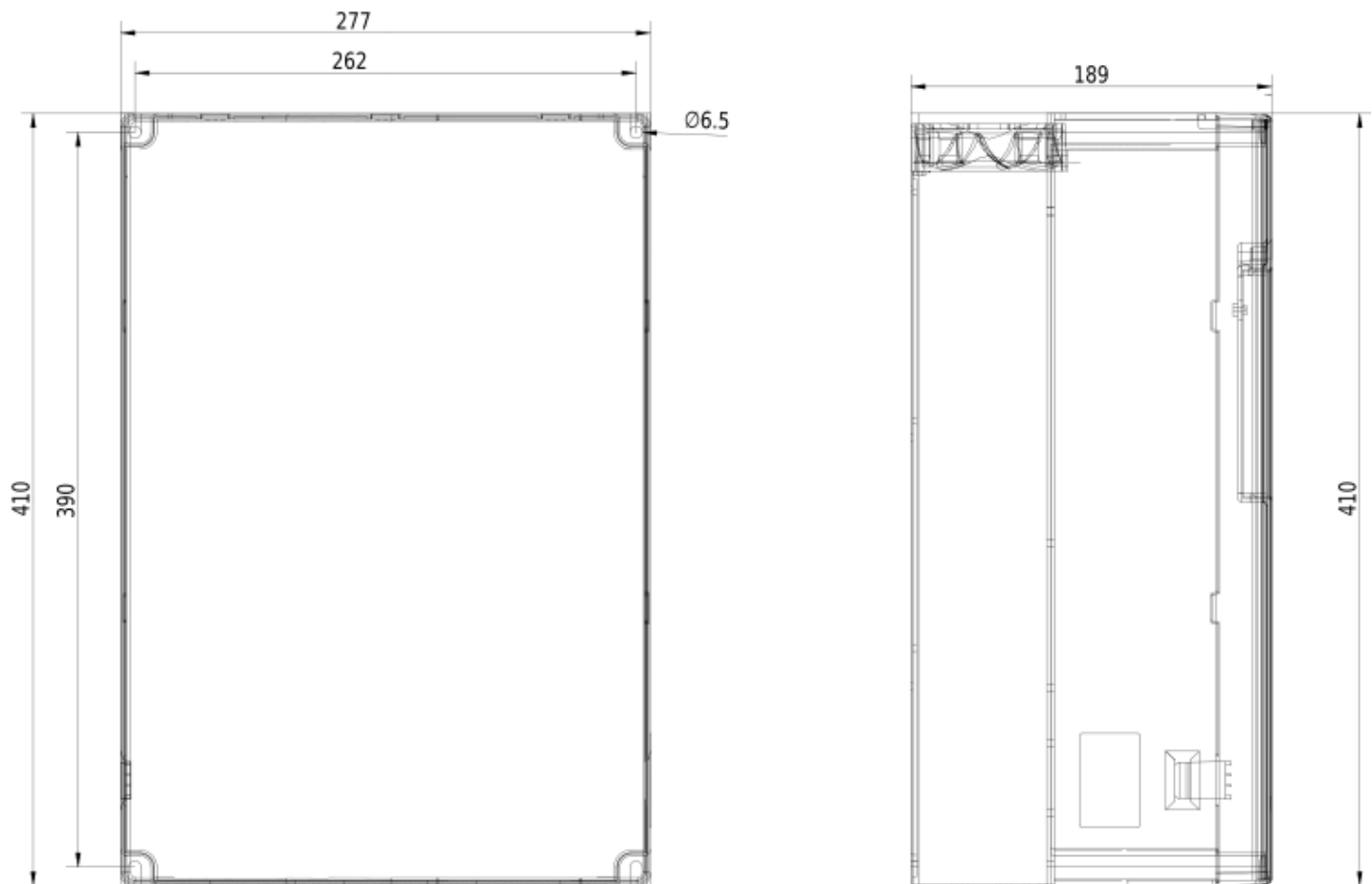
Rozmerový výkres V8 10 - 22kW 4T0220
