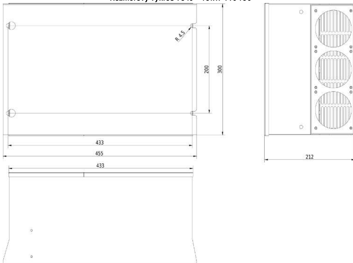
Rozmerový výkres V8 10 - 45kW 4T0450
