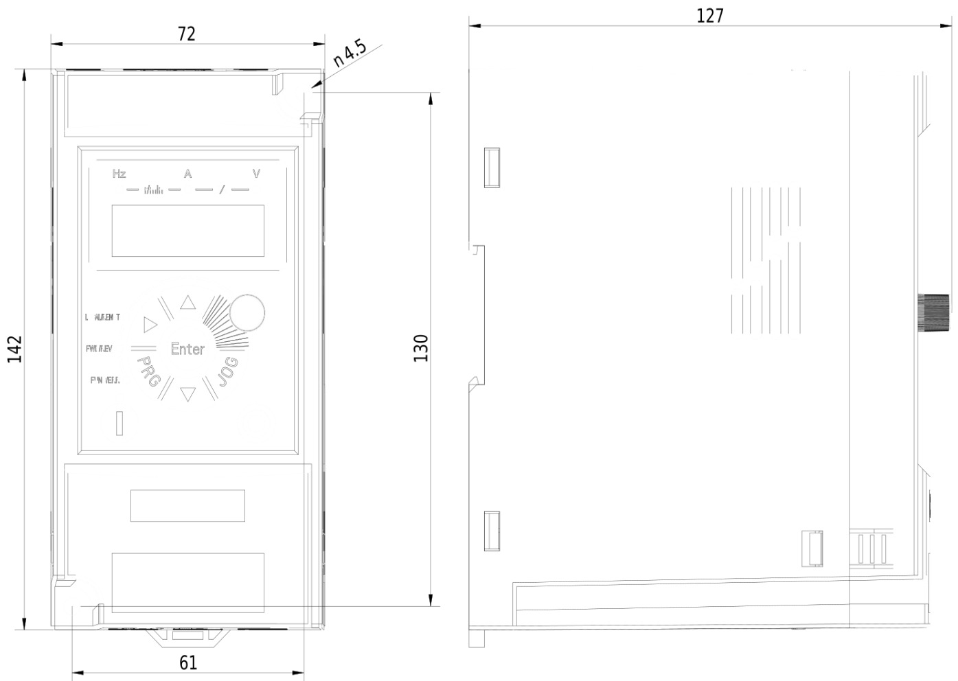
Rozmerový výkres V900 - 0,75kW 4T0007
