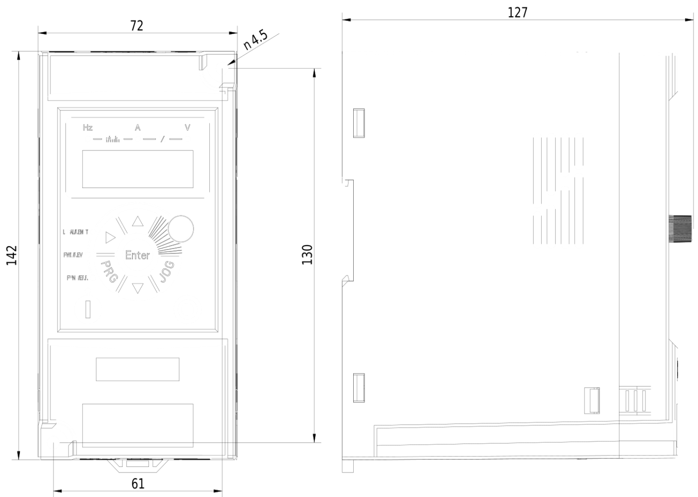
Rozmerový výkres V900 - 2,2kW 4T0022
