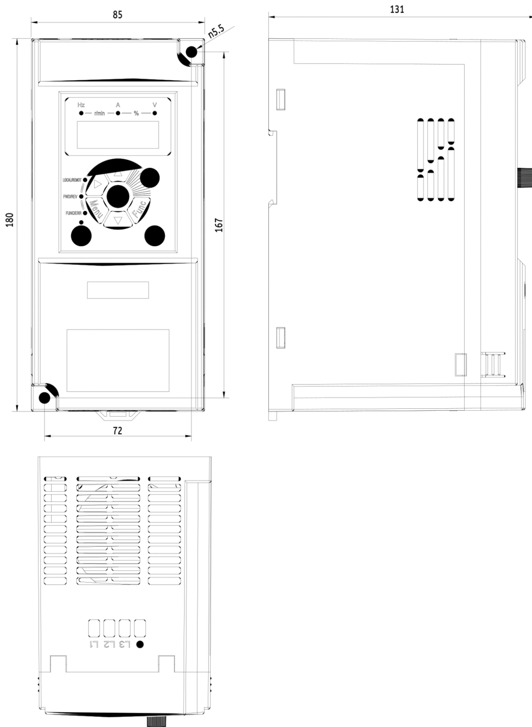
Rozmerový výkres V900 - 3,0kW 4T0030
