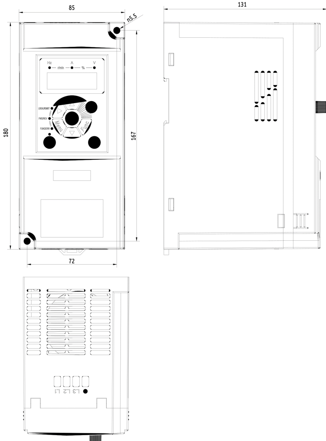
Rozmerový výkres V900 - 5,5kW 4T0055
