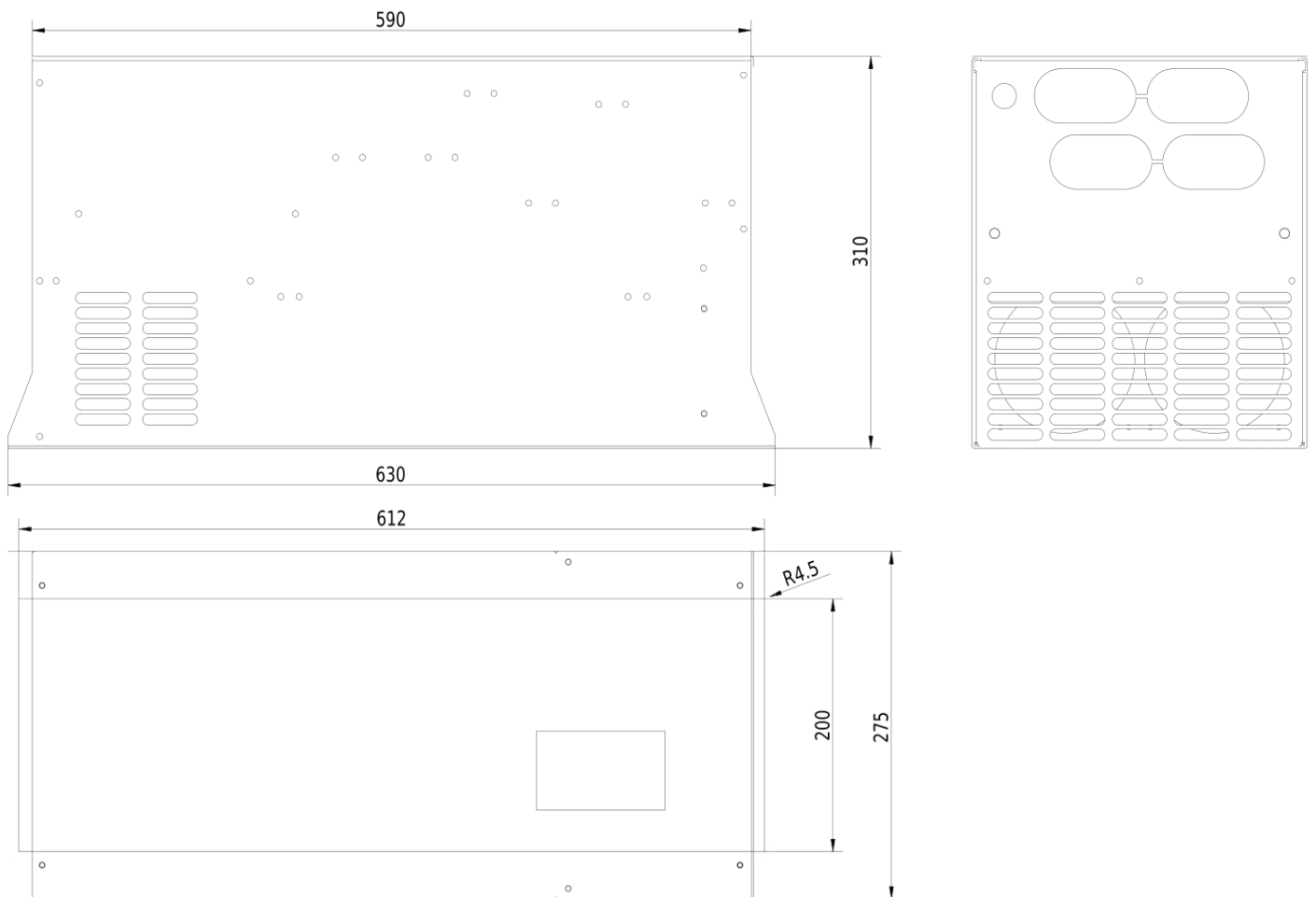
Rozmerový výkres V900 - 110kW 4T1100
