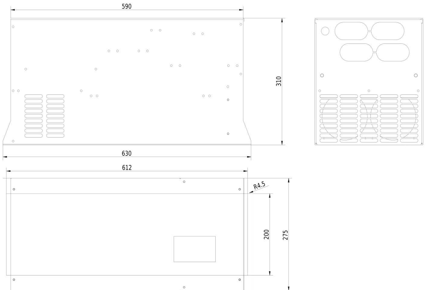
Rozmerový výkres V900 - 132kW 4T1320
