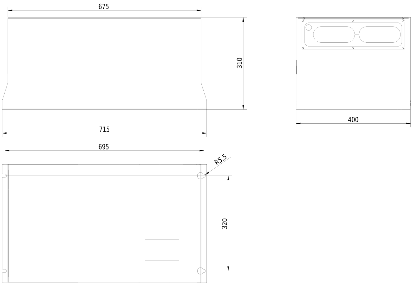
Rozmerový výkres V900 - 185kW 4T1850
