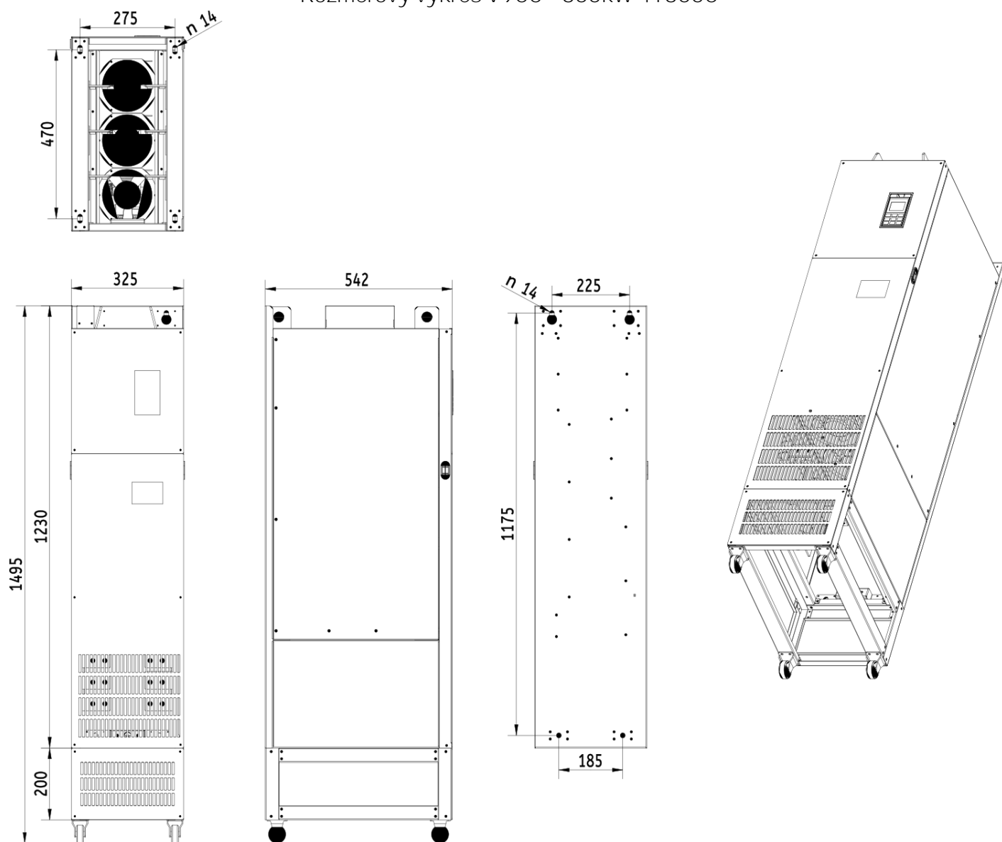
Rozmerový výkres V900 - 355kW 4T3550
