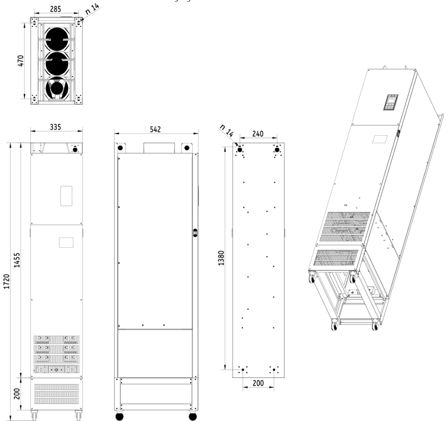
Rozmerový výkres V900 - 450kW 4T4500
